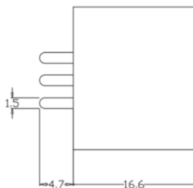
正视图
