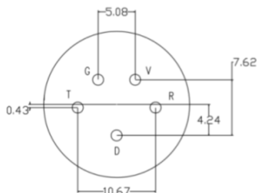
底视图
